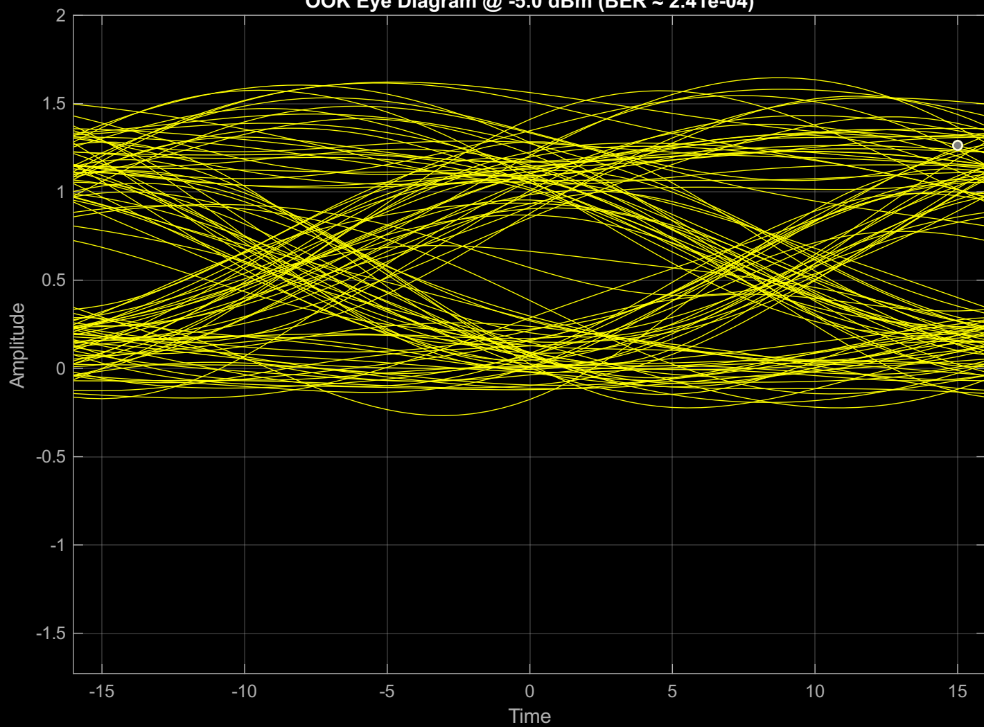
OOK Eye Diagram @ -5.0 dBm (BER \approx 2.41\text{e-}04 )
